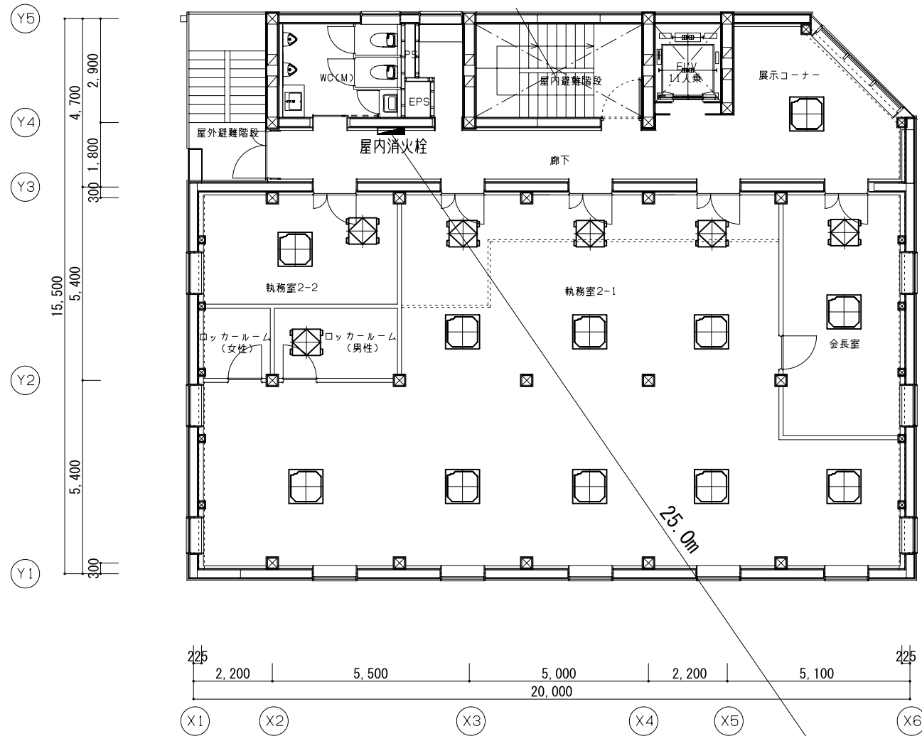
2F平面
