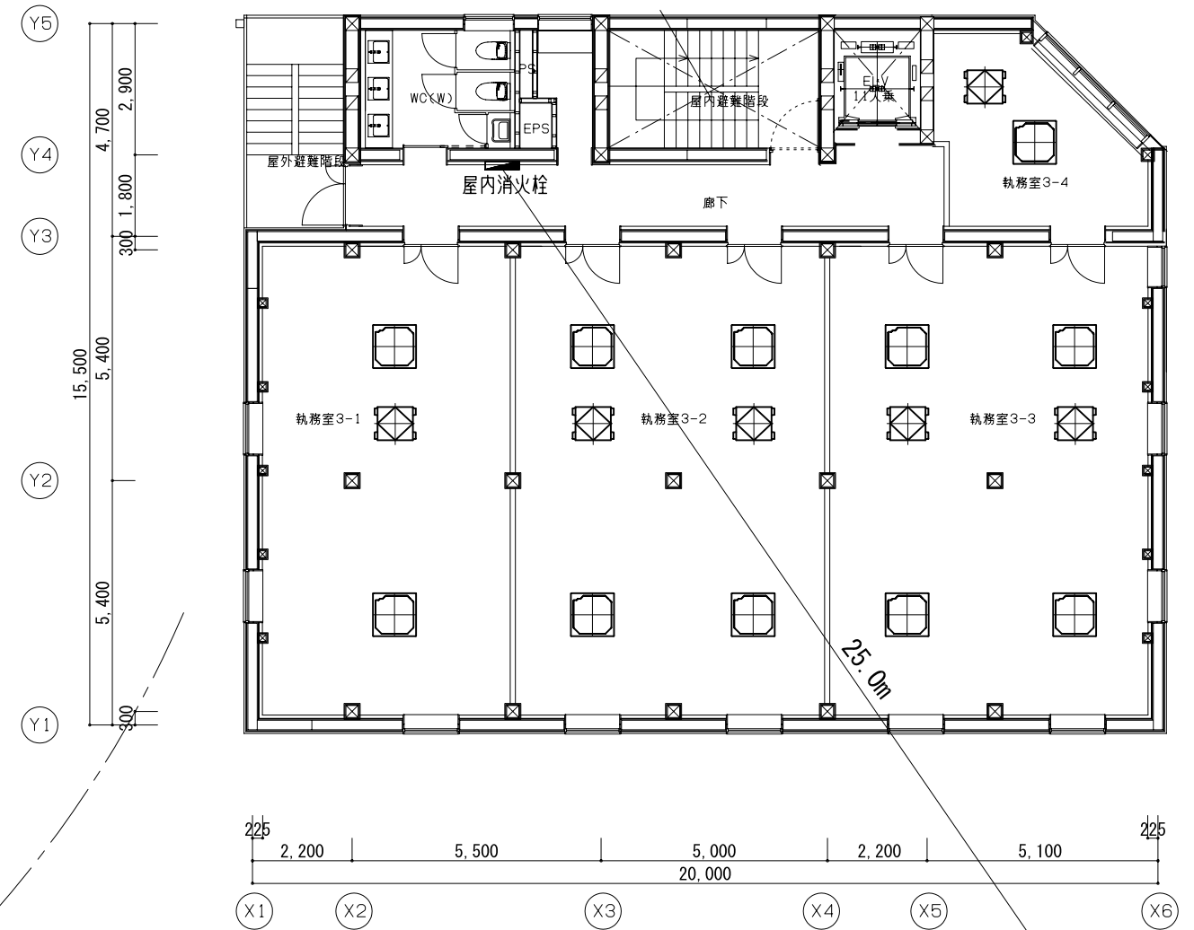
3F平面
