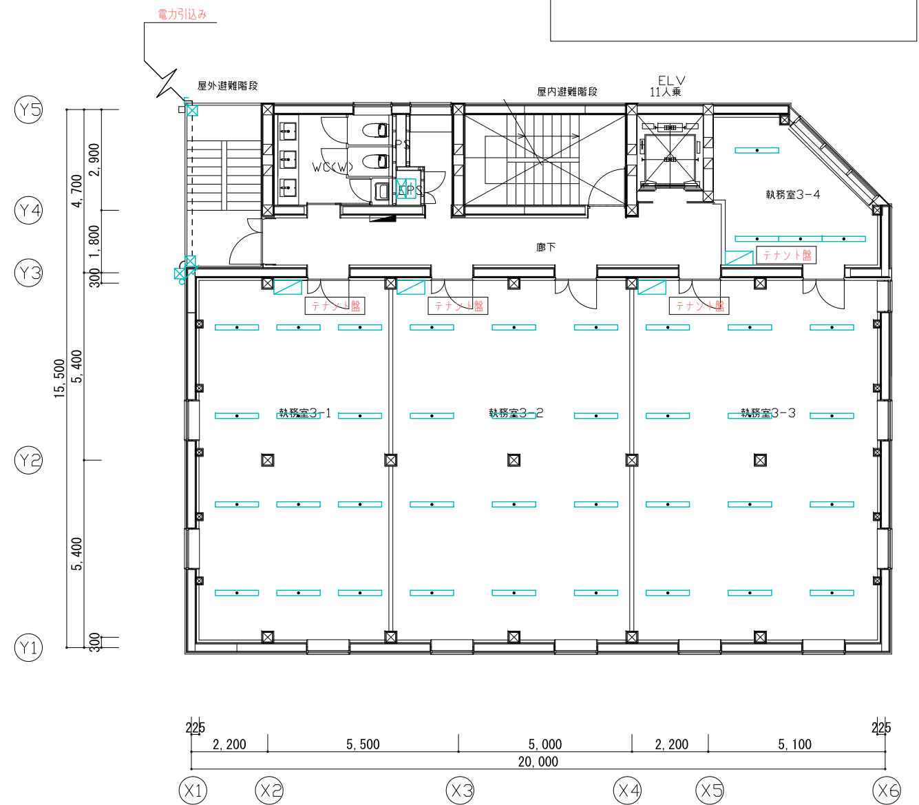
3F平面
