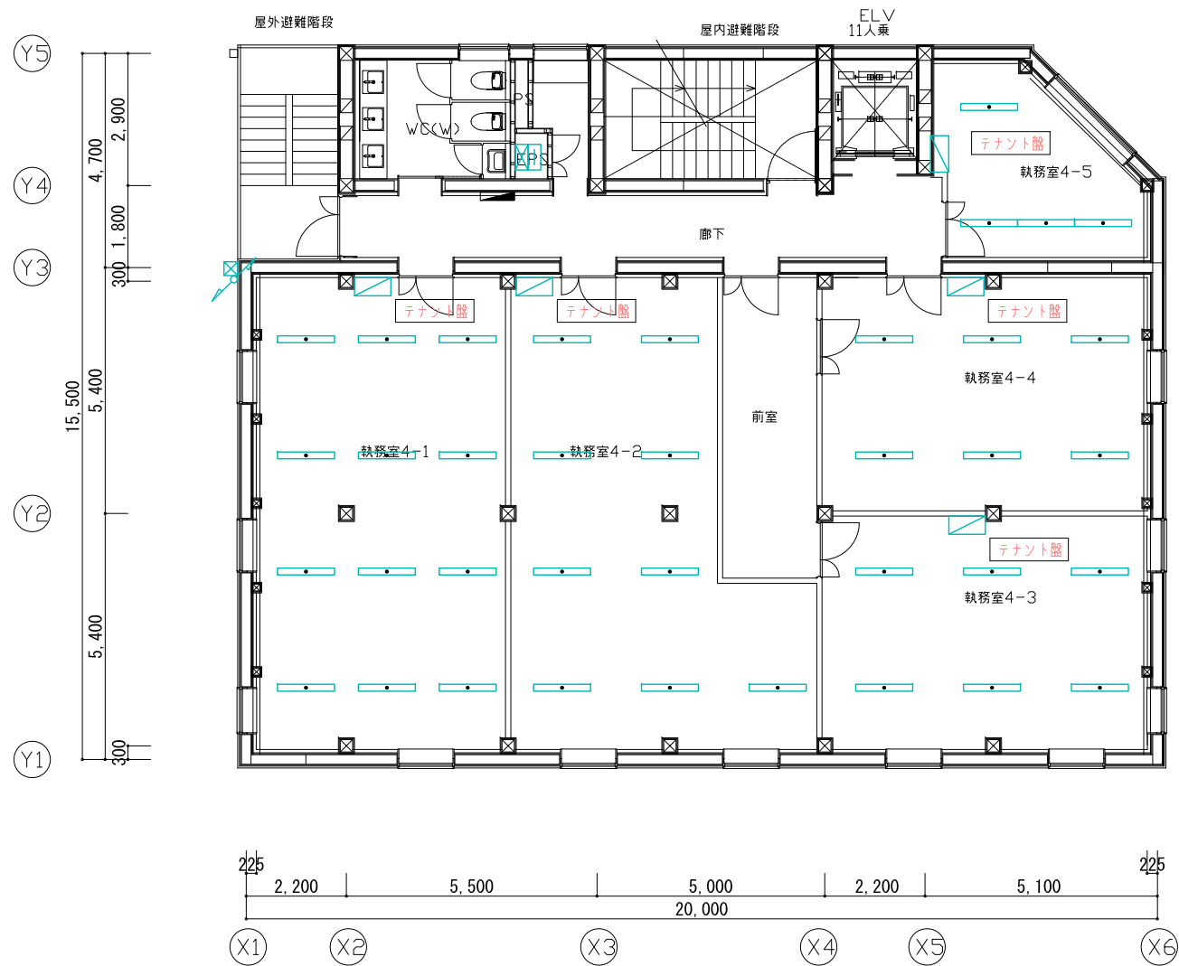
4F平面
