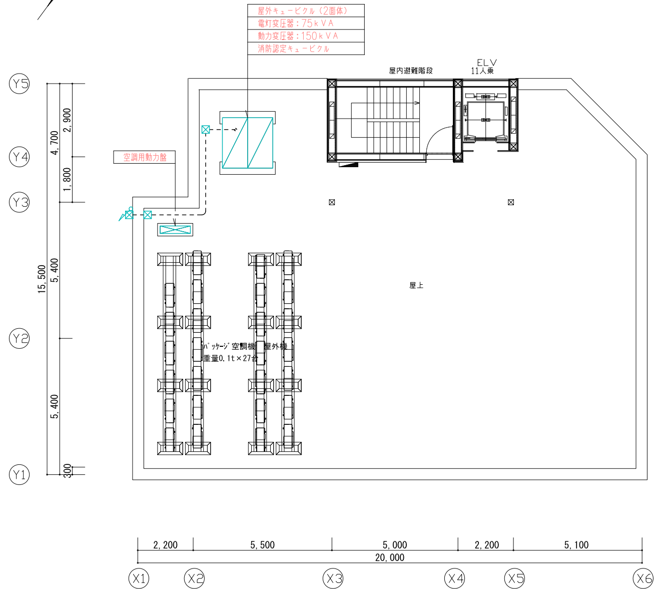
RF平面
