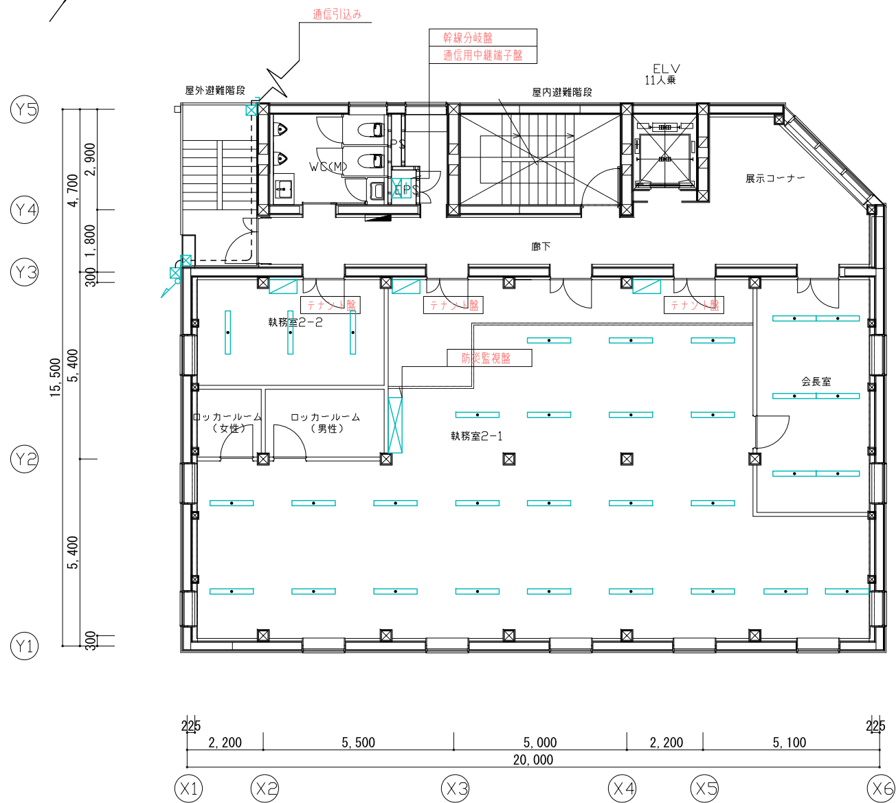
2F平面
