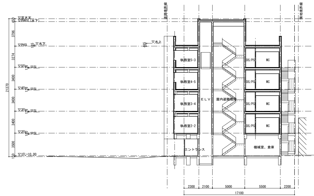
D-D断面図
