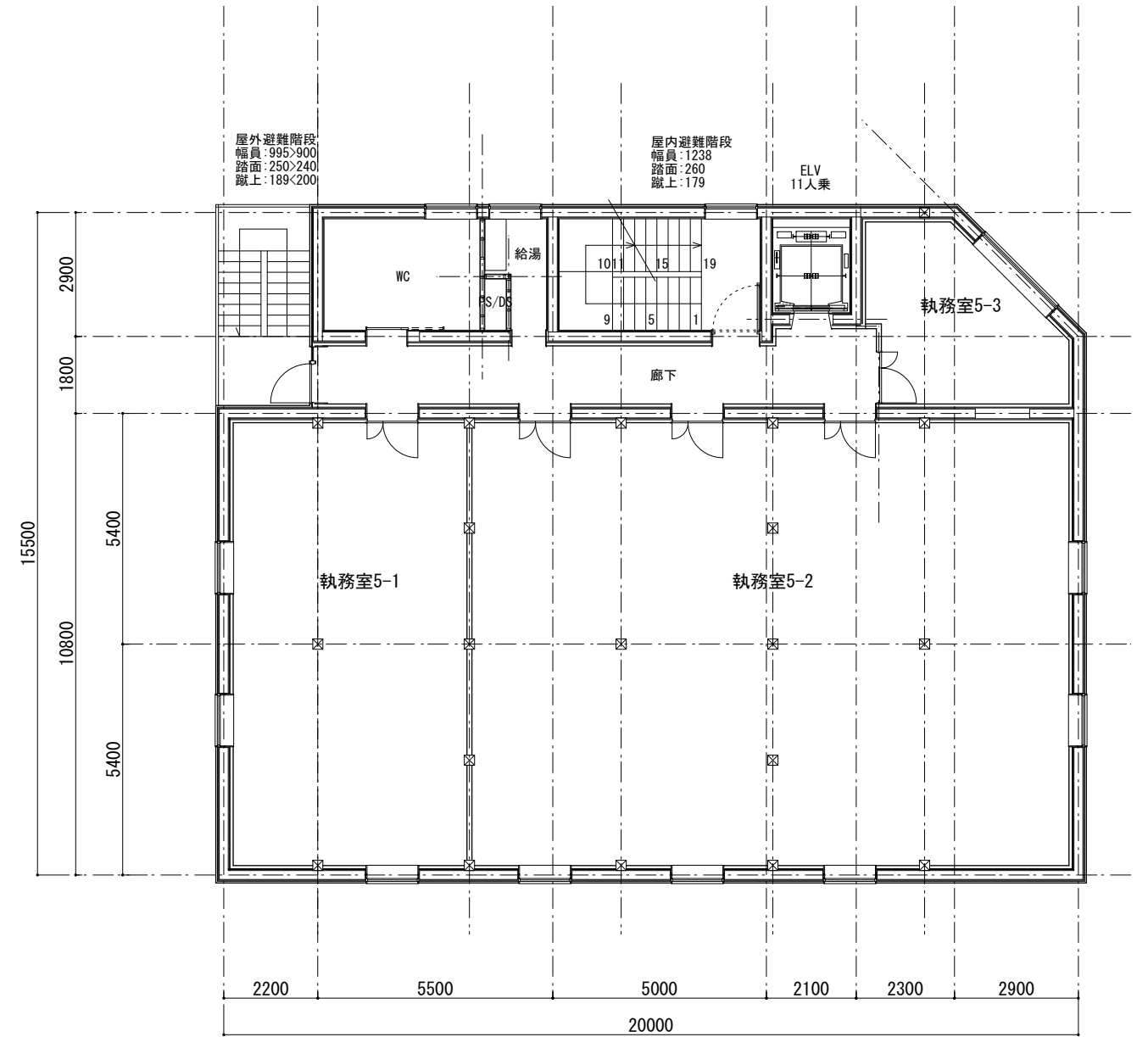
5F平面
