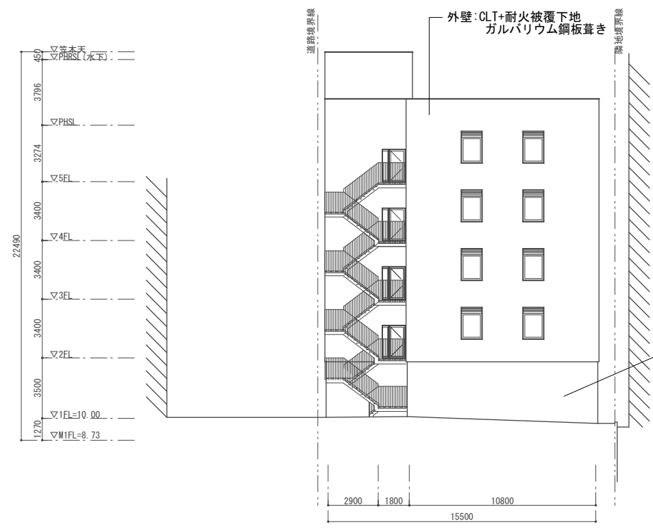
西立面図
