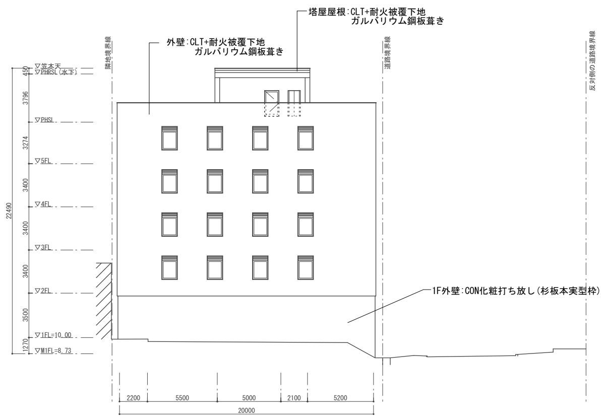
南立面図
