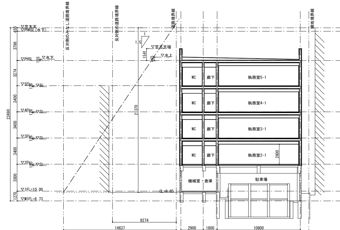
B-B断面図
