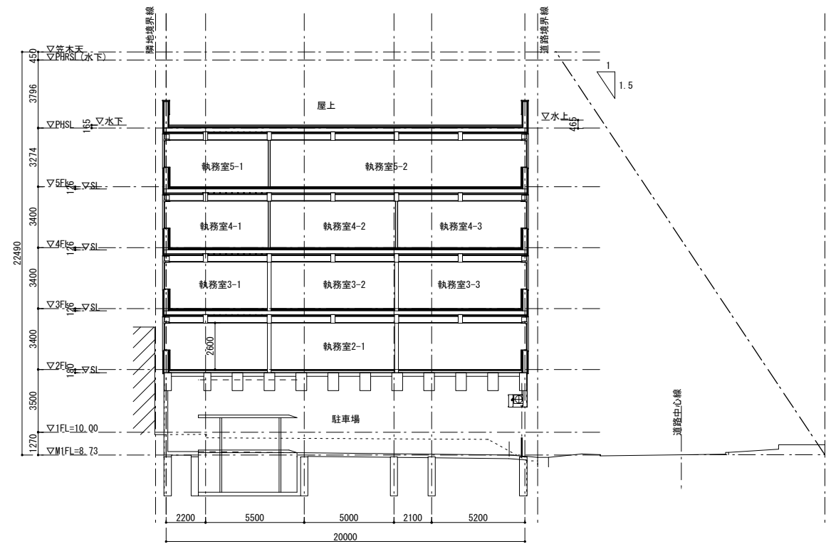
C-C断面図
