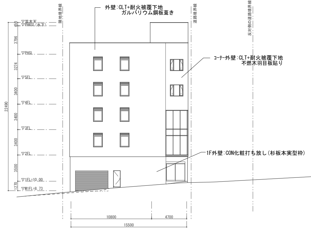
東立面図
