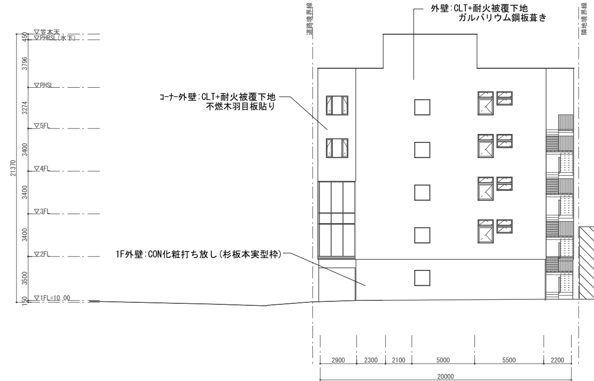
北立面図
