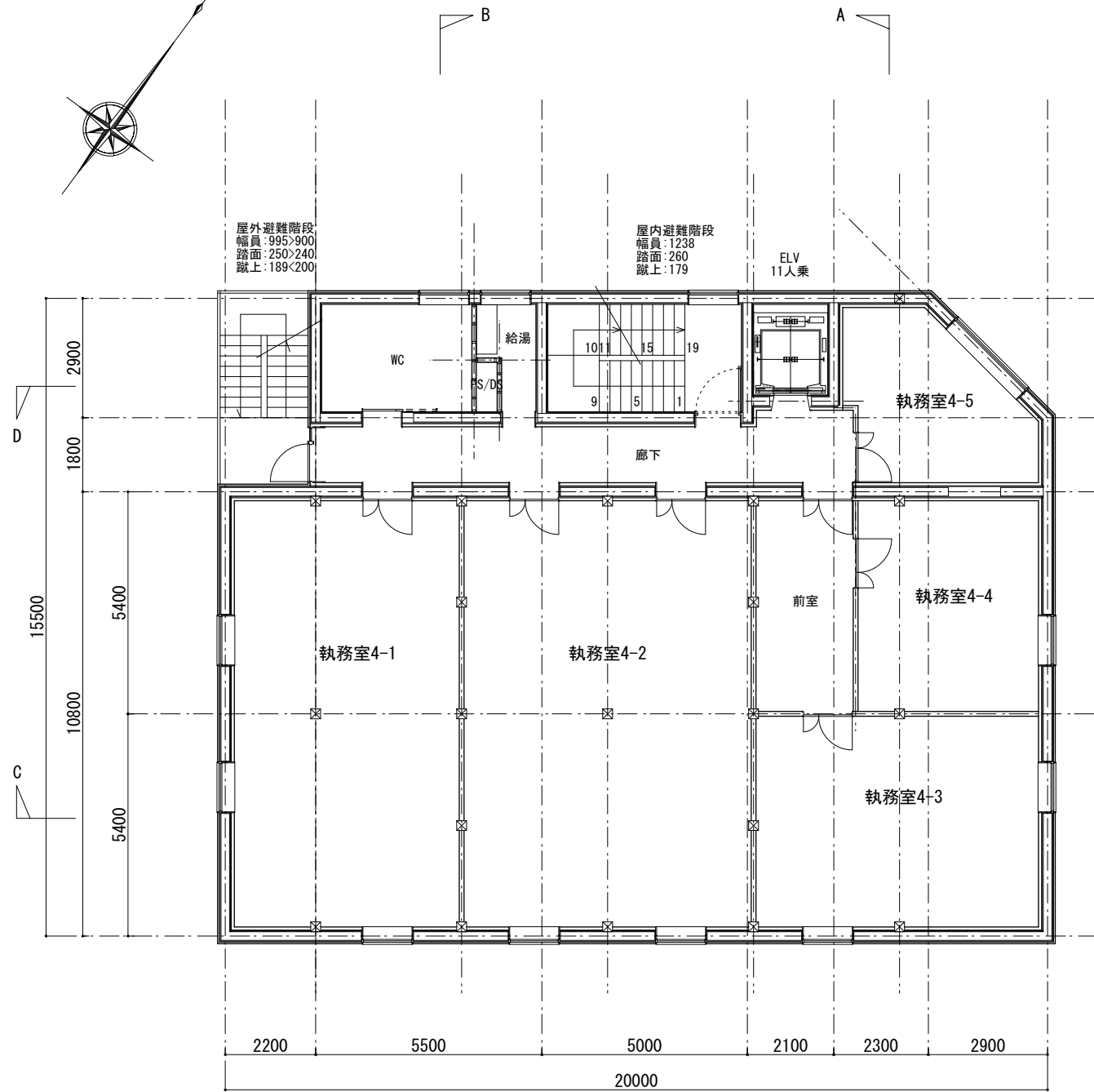
4F平面
