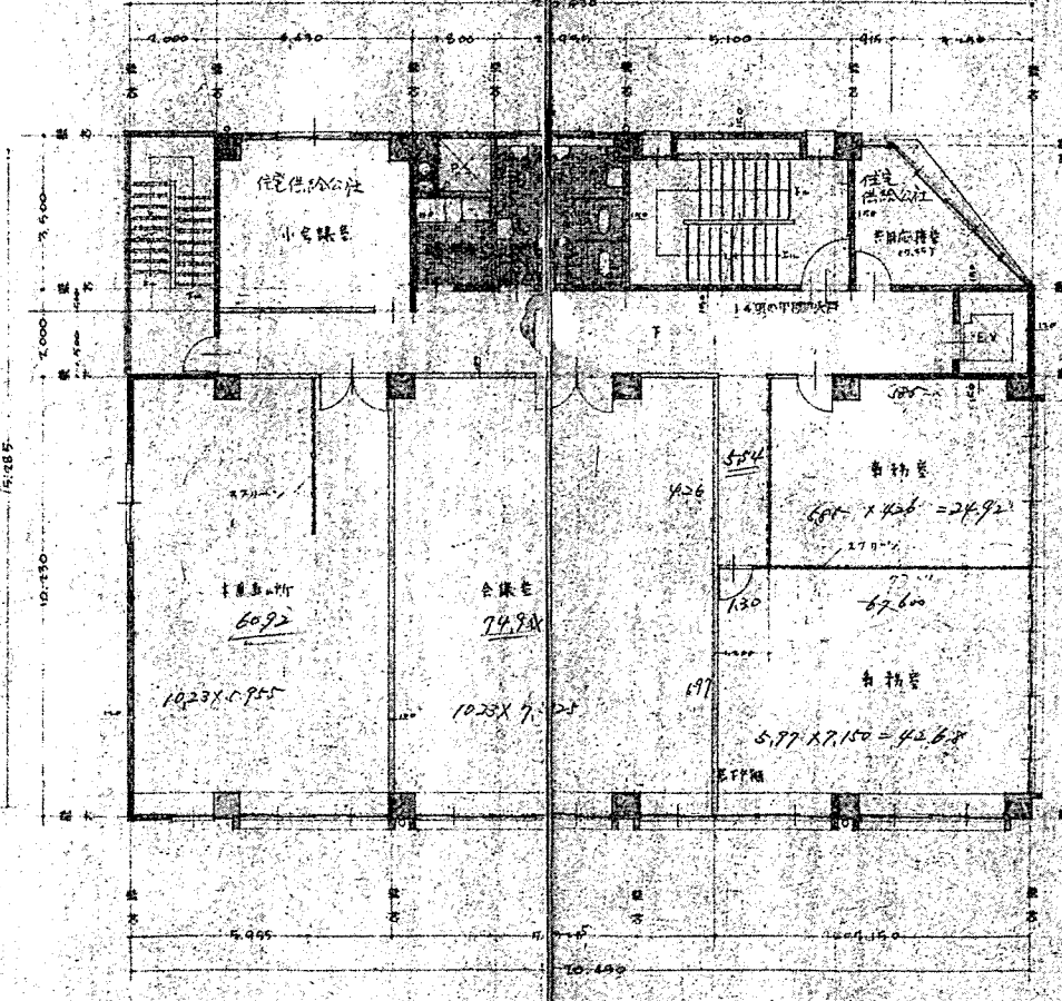
2階平面図 1:100
