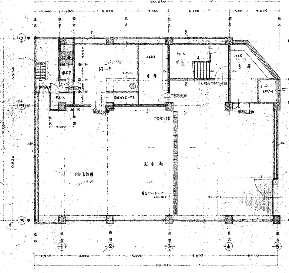
地階平面図 1:100
