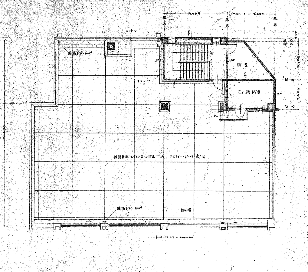
屋階平面図 1:100
