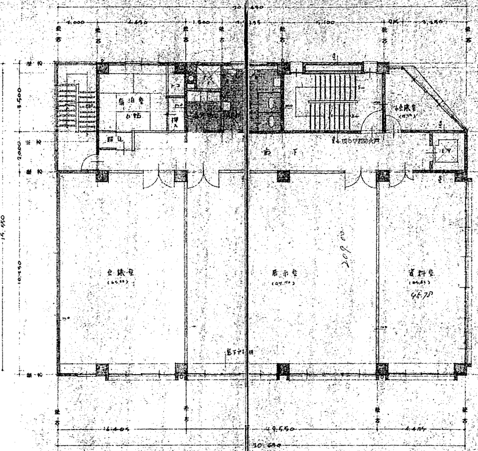
3階平面図 1:100
